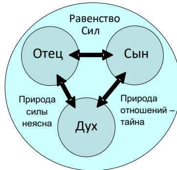
Модель Троица
