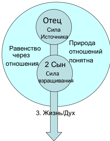
Модель Отец/Сын
